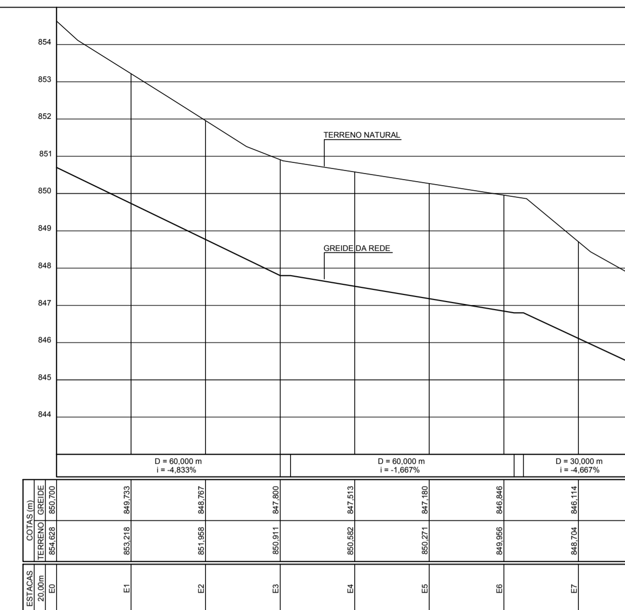
PERFIL LONGITUDINAL DO EIXO DA REDE ESCALA HORIZONTAL 1/000 ESCALA VERTICAL 1/00
