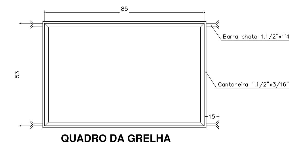
QUADRO DA GRELHA ESCALA 1:10
