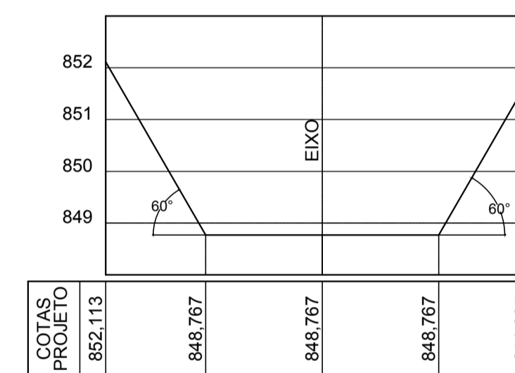
CORTE TRANSVERSAL EST. 2 ESCALA 1/100
