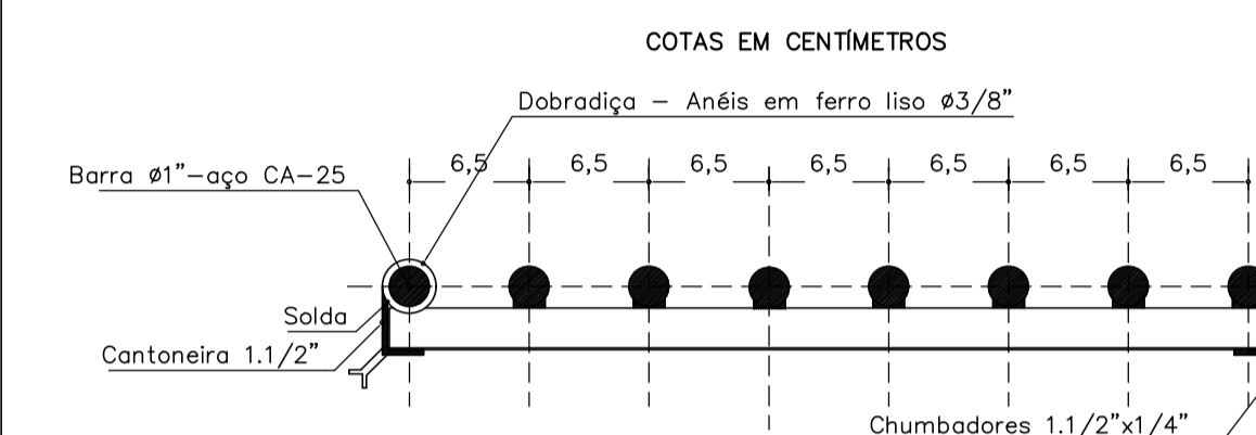
CORTE AA - BERÇO DA GRELHA ESCALA 1:5
