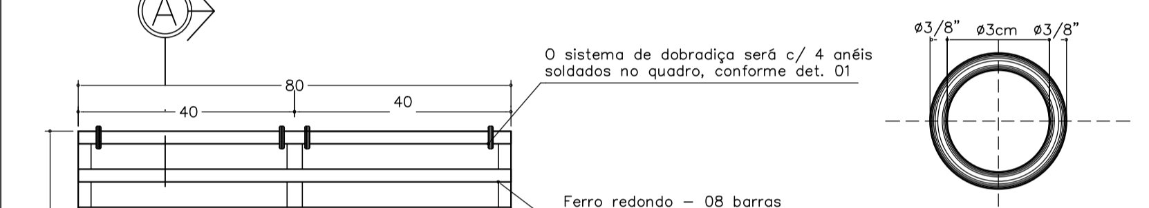
DETALHE 01 - (ANÉIS) SEM ESCALA
